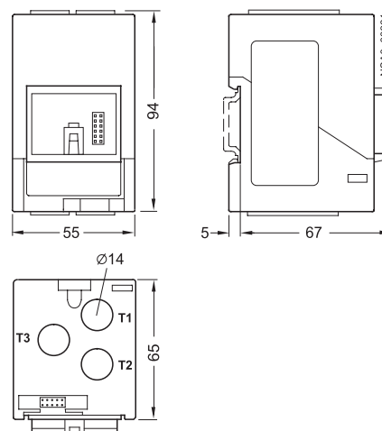
电流检测模块 (穿芯式) 3UF7 103
