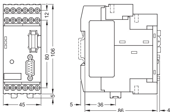
SIMOCODE pro C 基本单元, 3UF7 000
