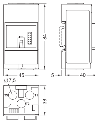
电流检测模块 (穿芯式) 3UF7 102
