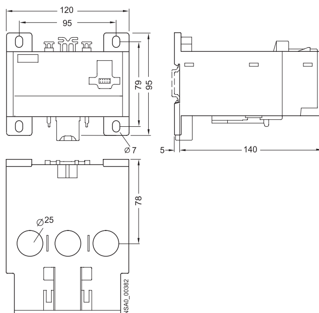
电流检测模块 (穿芯式) 3UF7 103
