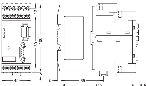
SIMOCODE pro V 基本单元, 3UF7 010
