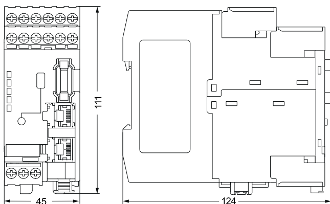
SIMOCODE pro V 基本单元 (PROFINET), 3UF7 011
